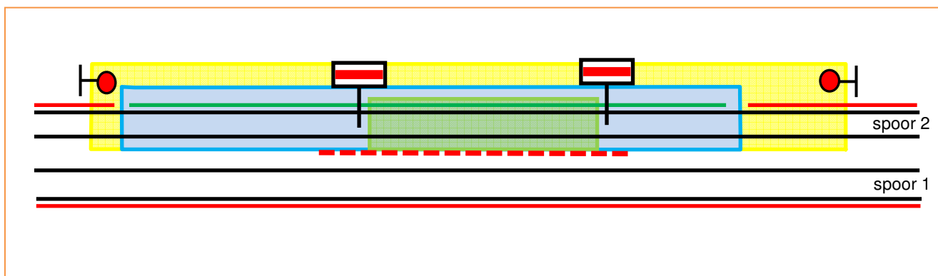
Figuur 5. Voorbeeld van veiligheidsschillen bij werkplek op een enkelsporig buiten dienst gesteld spoor.
