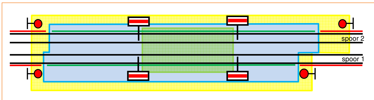
Figuur 4. Voorbeeld van veiligheidsschillen bij werkplek op een dubbelsporig buiten dienst gesteld spoor.
