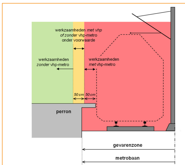
Figuur 10. Werkzaamheden op het perron van een bovengronds traject.
