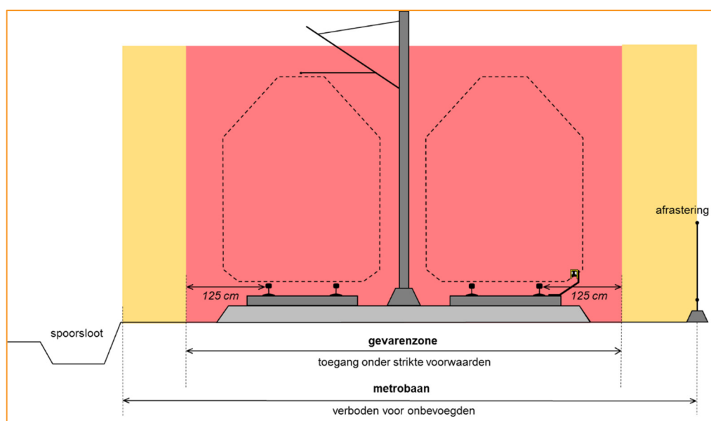
Figuur 7. Voorbeeld van de metrobaan met de gevarenzone op een bovengronds traject.
