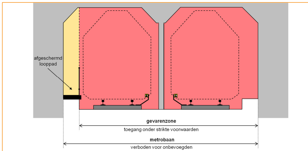
Figuur 9. Gevaarzone in de tunnel met afgeschermd looppad.
