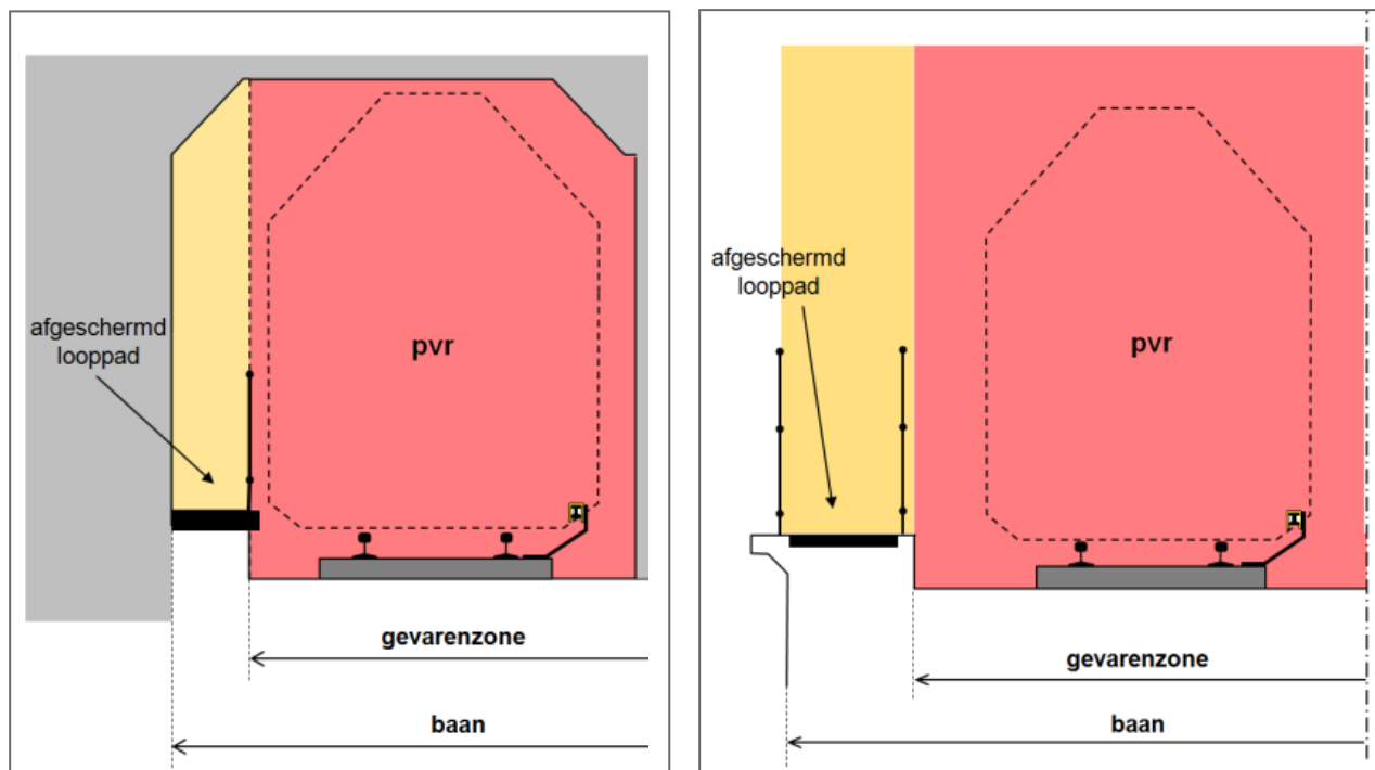
Figuur 8: Voorbeelden van een afgeschermd looppad in de tunnel en op viaduct.
