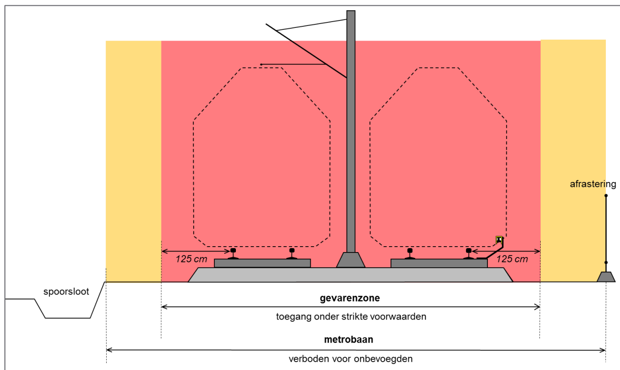
Figuur 4: Voorbeeld van de baan met de gevarenszone op een bovengronds traject.
