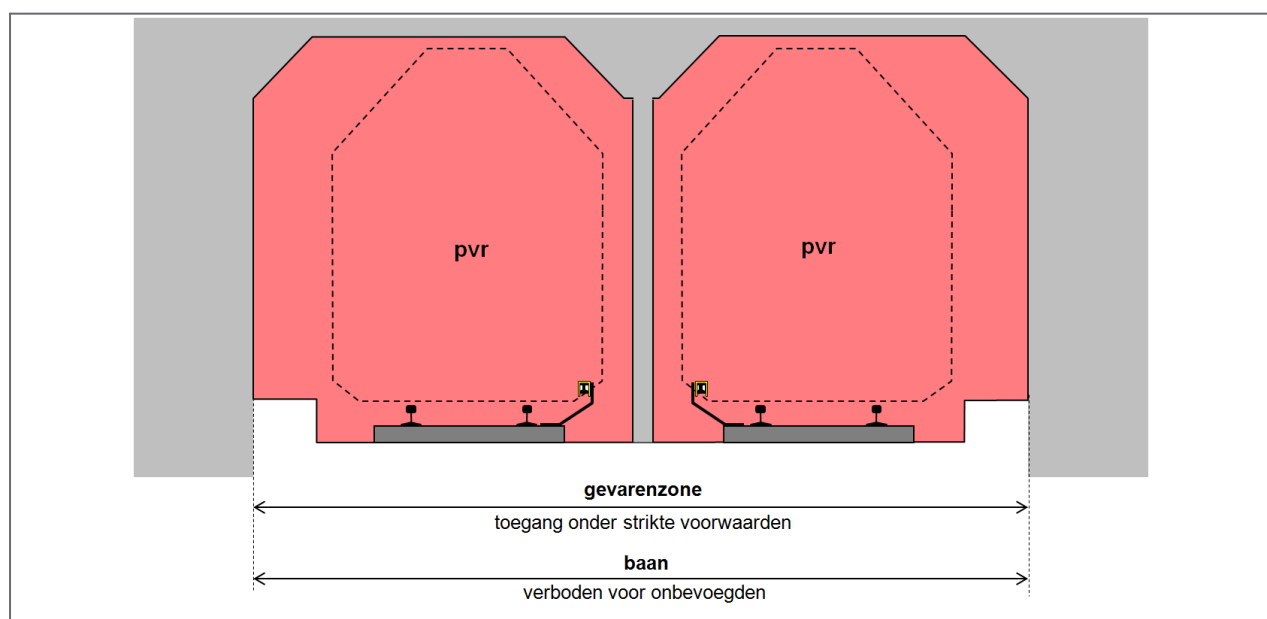
Figuur 5: Voorbeeld van de baan met de gevarenszone in een tunnel.
