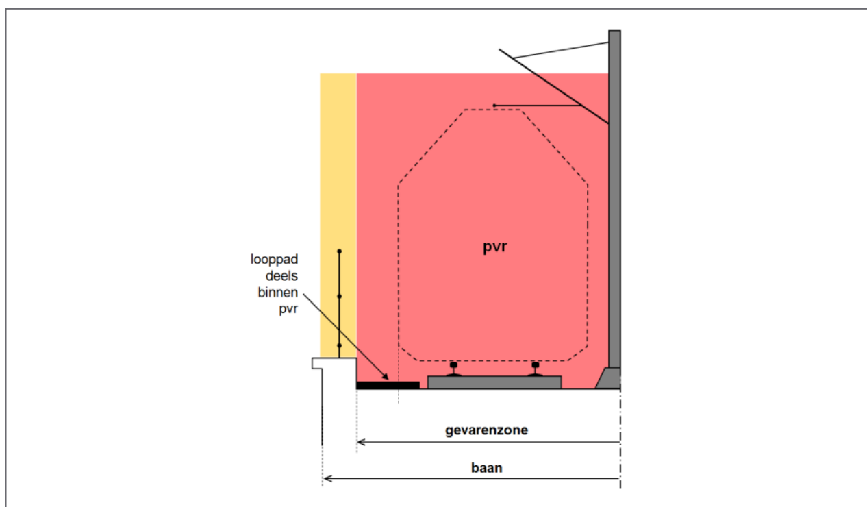
Figuur 7: Voorbeeld van looppad deels binnen pvr.
