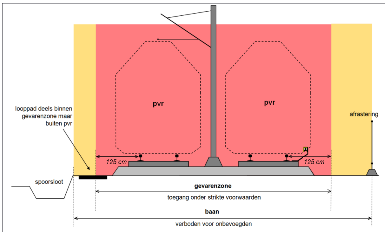
Figuur 6: Voorbeeld van looppad binnen gevarenczone, maar buiten pvr.
